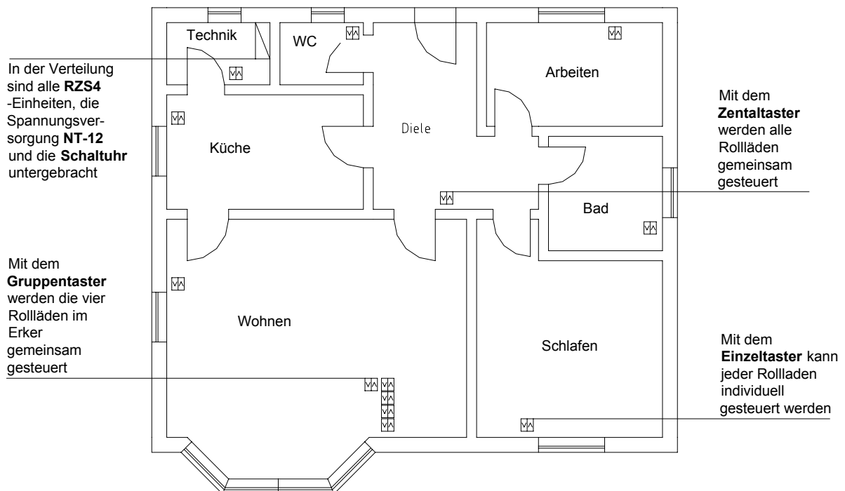
Beispiel einer Zentralsteuerung in einem Einfamilienhaus
