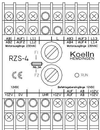
Eine RZS-4-Einheit
